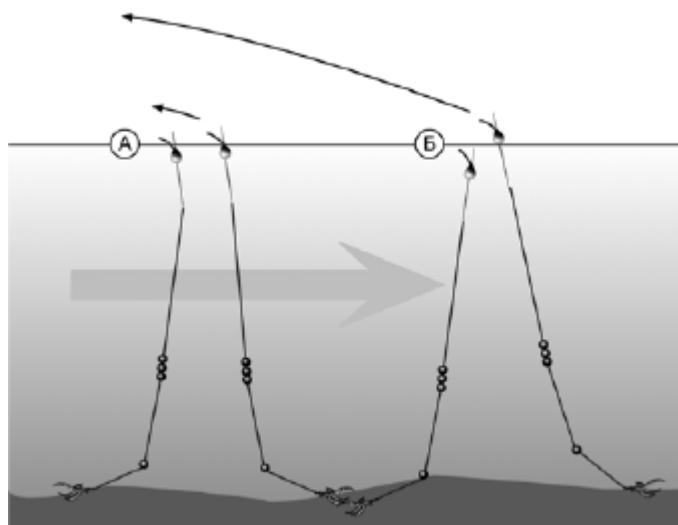
Рис. 53. Манипуляции со снастью при проводке
