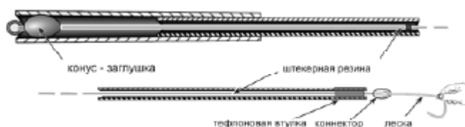
Рис. 56. Схема амортизатора
