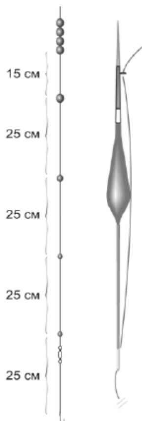
Рис. 45. Оснастка для ловли в медленно текущей воде
